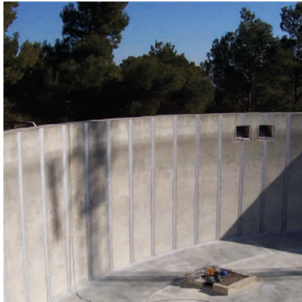
Réservoir Dupail, France: 900 m of Sikadur® Combiflex® SG Tapes.
