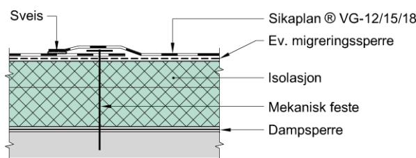
Fig. 1 Eksempel på mekanisk feste av Sikaplan® VG PVC takbelegg i banekant.
