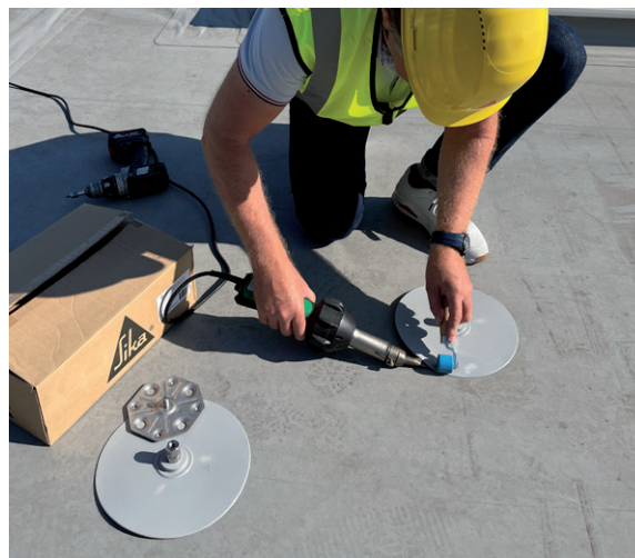
Mansjett blir montert på festebraketten og varmluftsveises på takbelegget.
