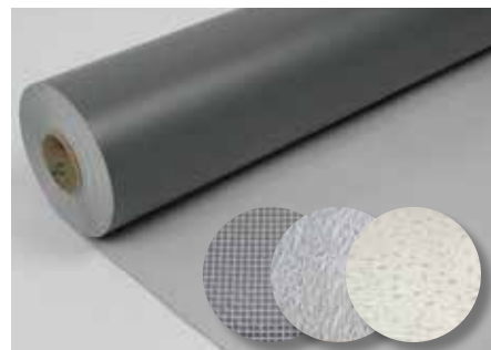
Sikaplan® U-15 TEX er en flerlags polyester og glassfiberforsterket PVC-membran. Produktet er egnet på eksponerte og ballasterte tak, samt grønne tak.
