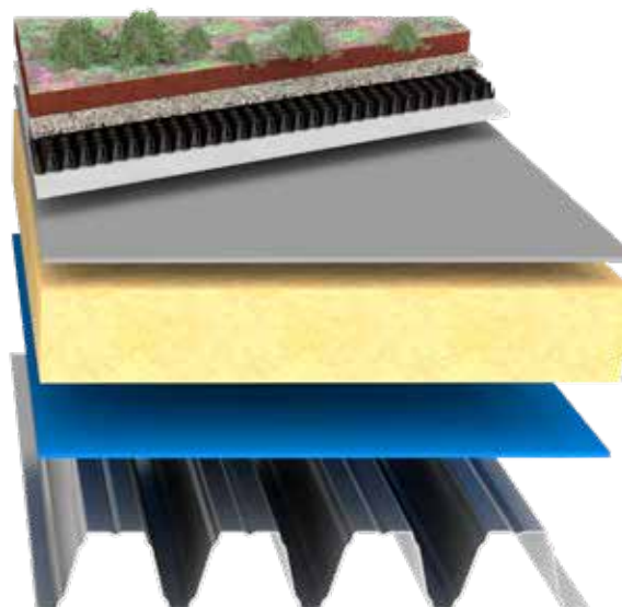
Ballastert tak
