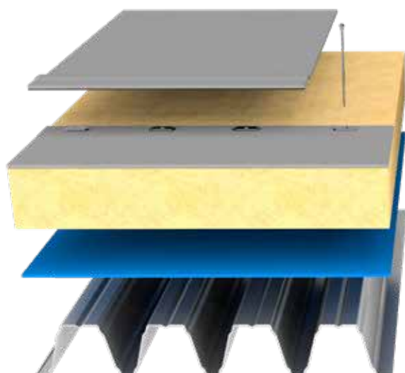
Kompakt tak
